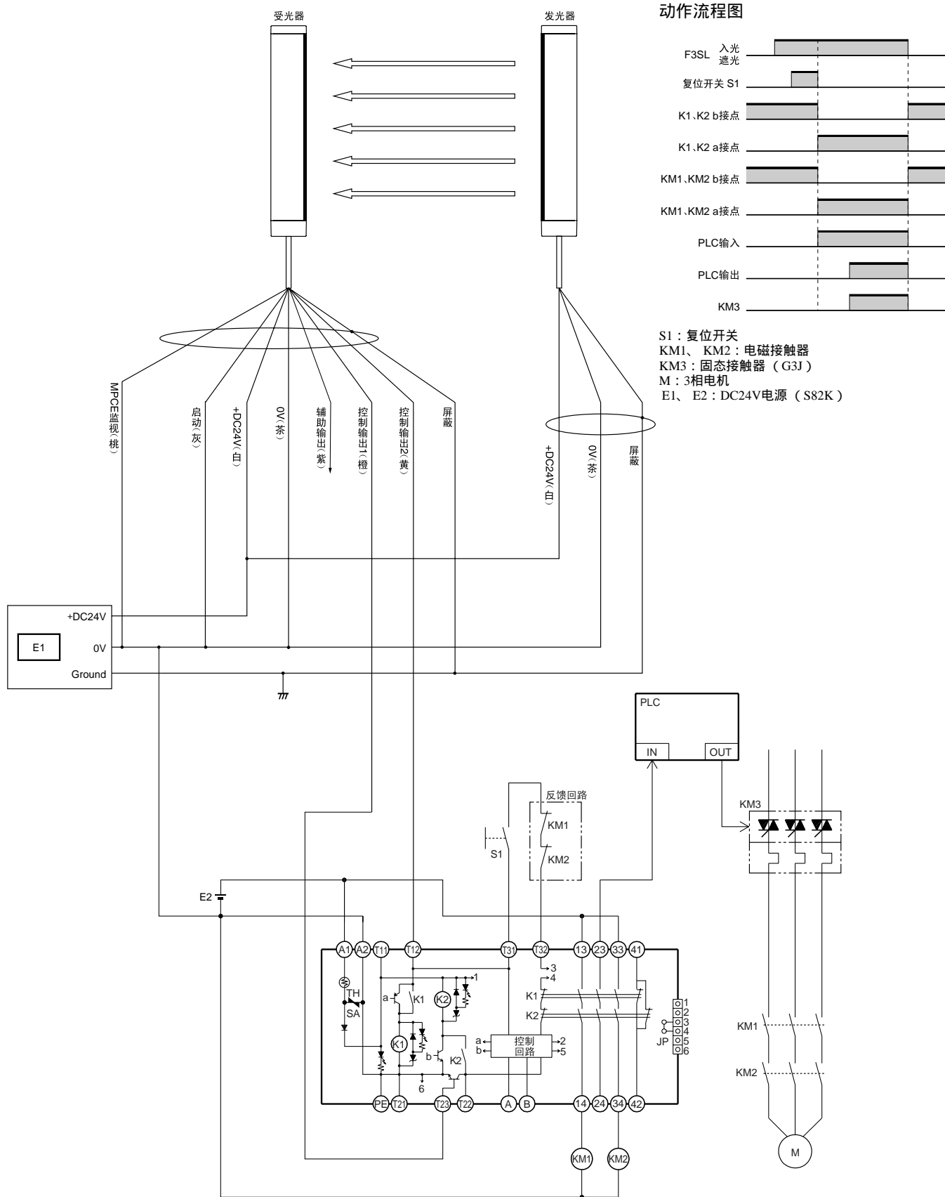
动作流程图
