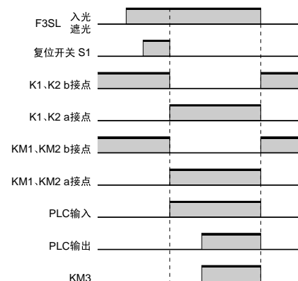
动作流程图
