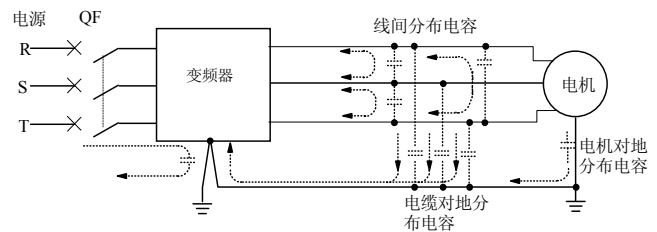
图3-42 漏电流路径
